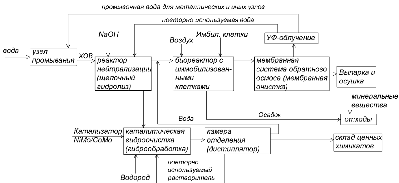
Рис. 1. Блок-схема очистки сточных вод завода по уничтожению химического оружия в Удмуртии
