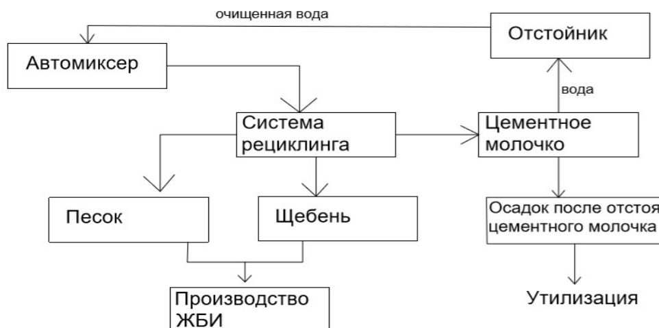
Рис.2. Технология рециклинга бетонной смеси
