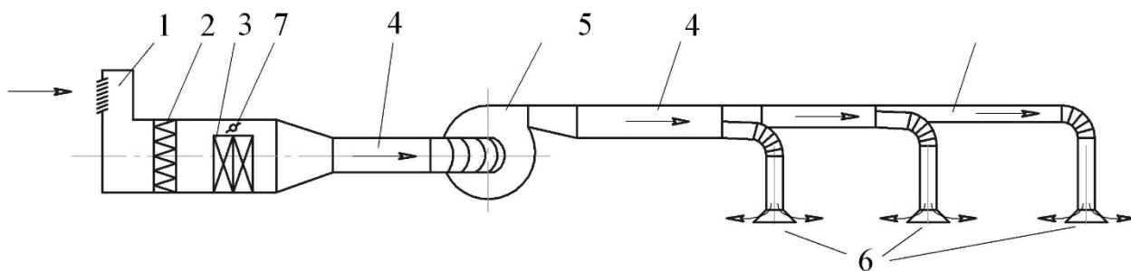
Рисунок 1. Схема вентиляции воздуха
