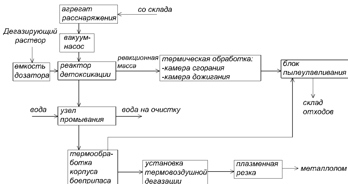
Рис. 1. Технологическая схема уничтожения химического оружия методом детоксикации в реакторе
